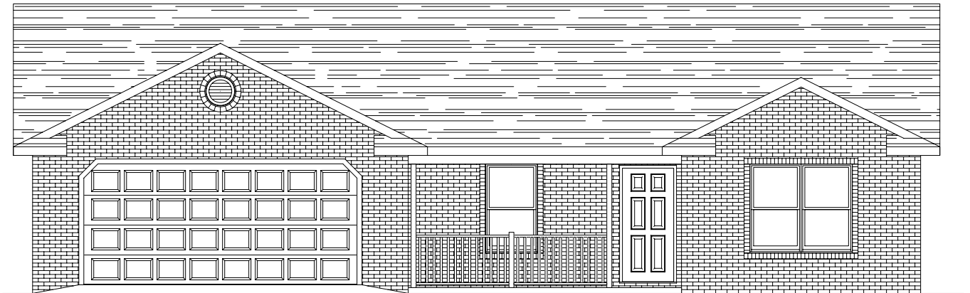
ELEVATION "C"
